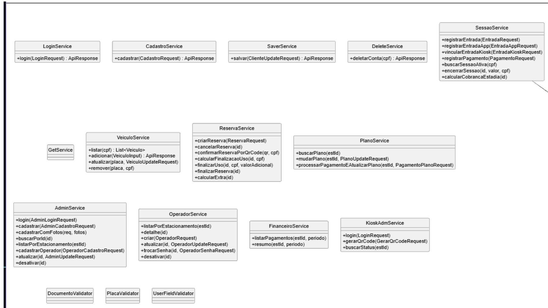
Figura 40 - C4 Nível 4 - Services (1/2)
