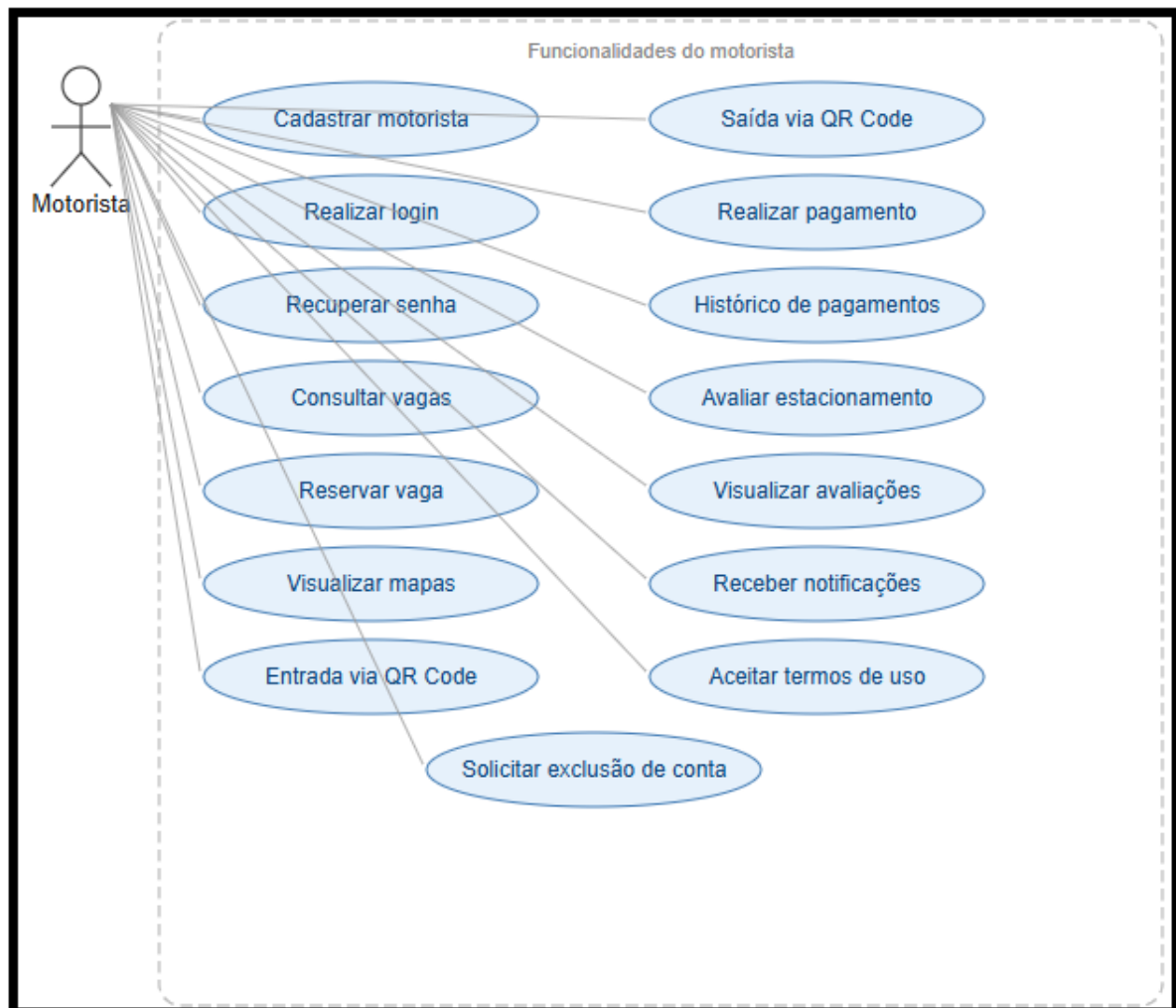
Figura 6 - Diagrama de casos de uso - Parte 1
