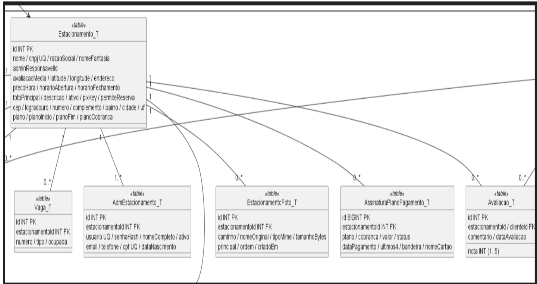
Figura 50 - C4 Nível 4 - Integrações com o banco de dados (2/2)
