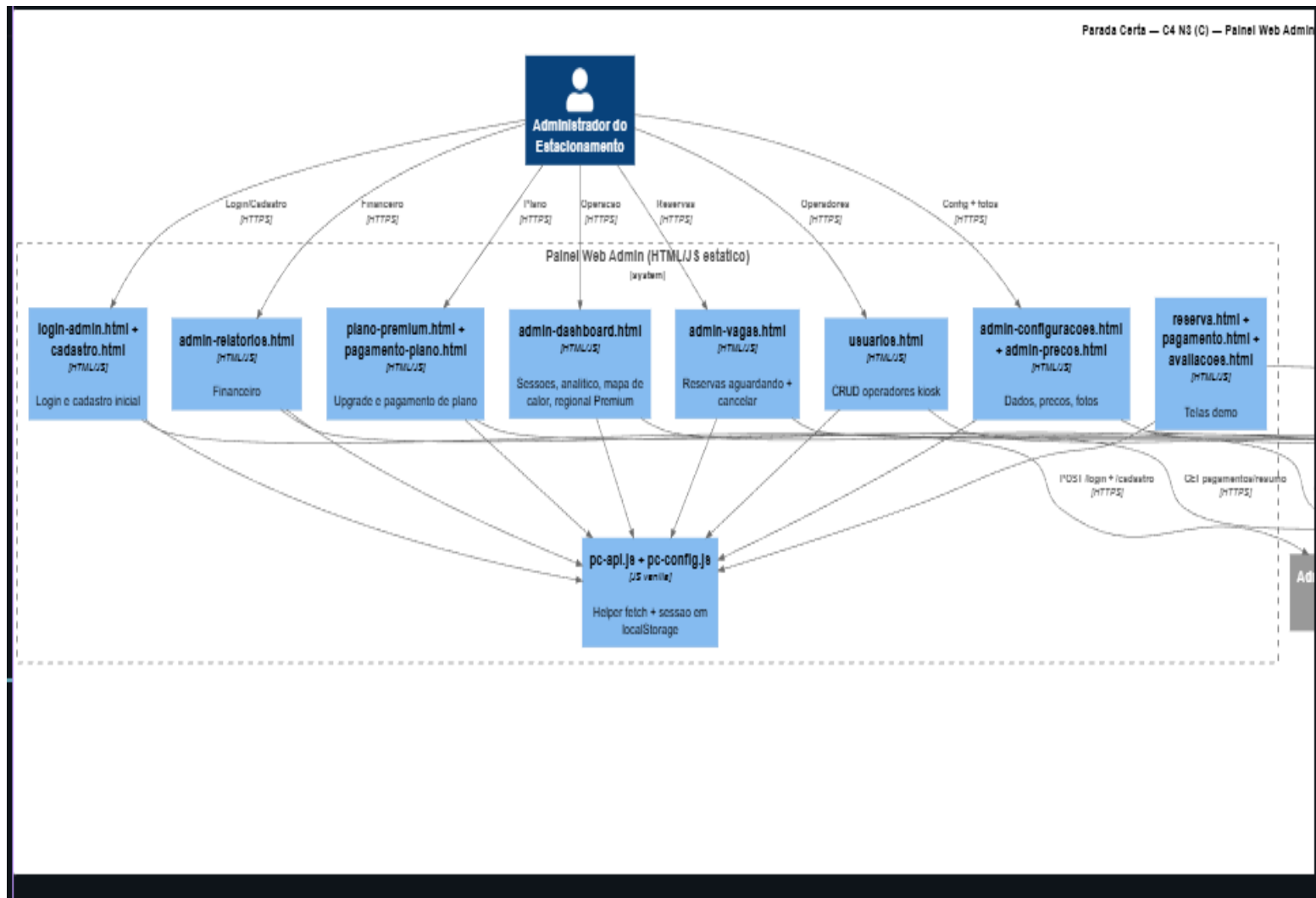
Figura 33 - C4 Nível 3 - Web
