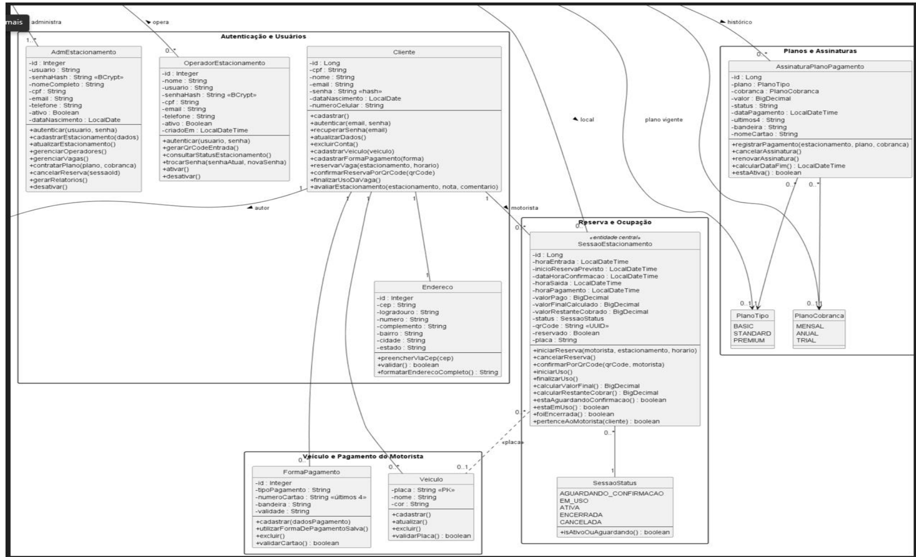
Figura 11 - Diagrama de classes separado - (2/2)
