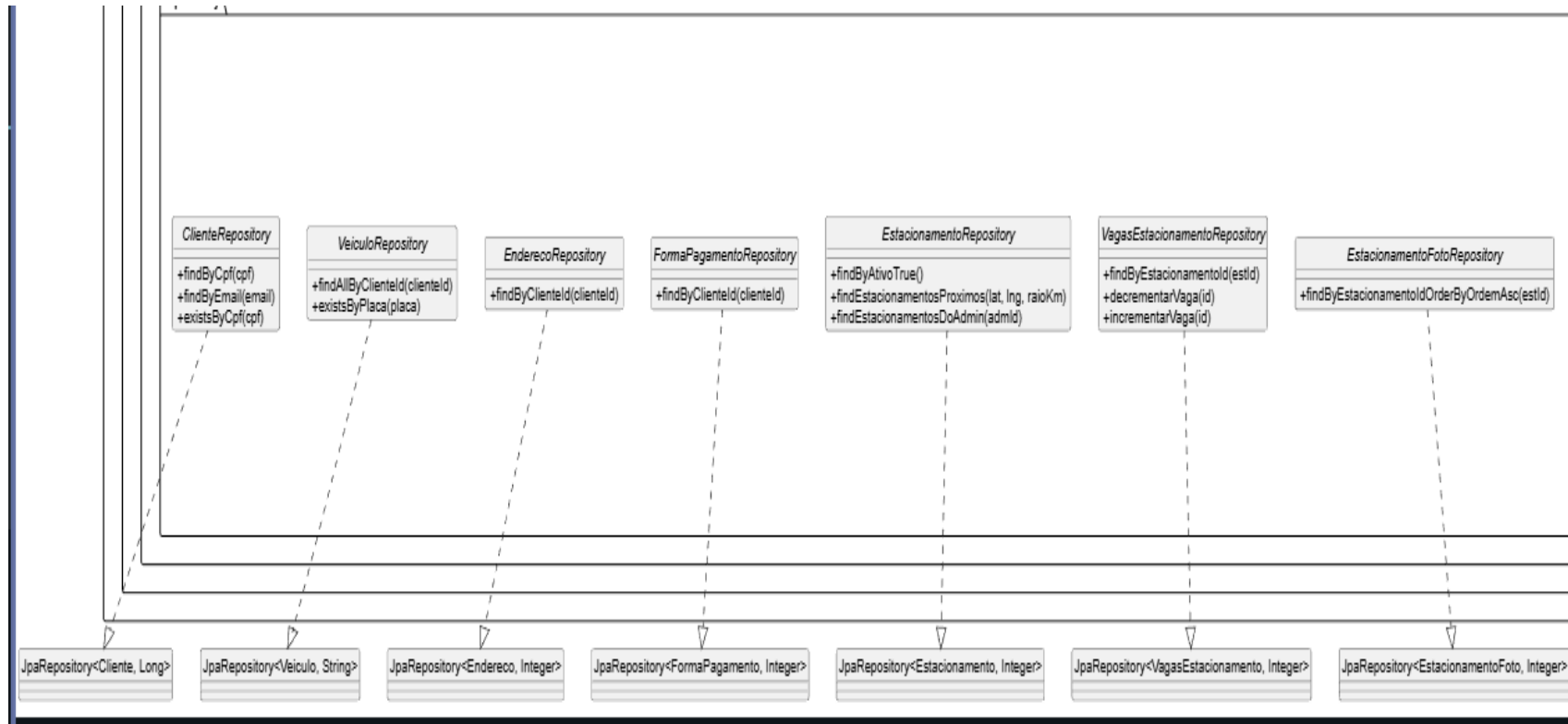
Figura 42 - C4 Nível 4 - Repository (1/3)
