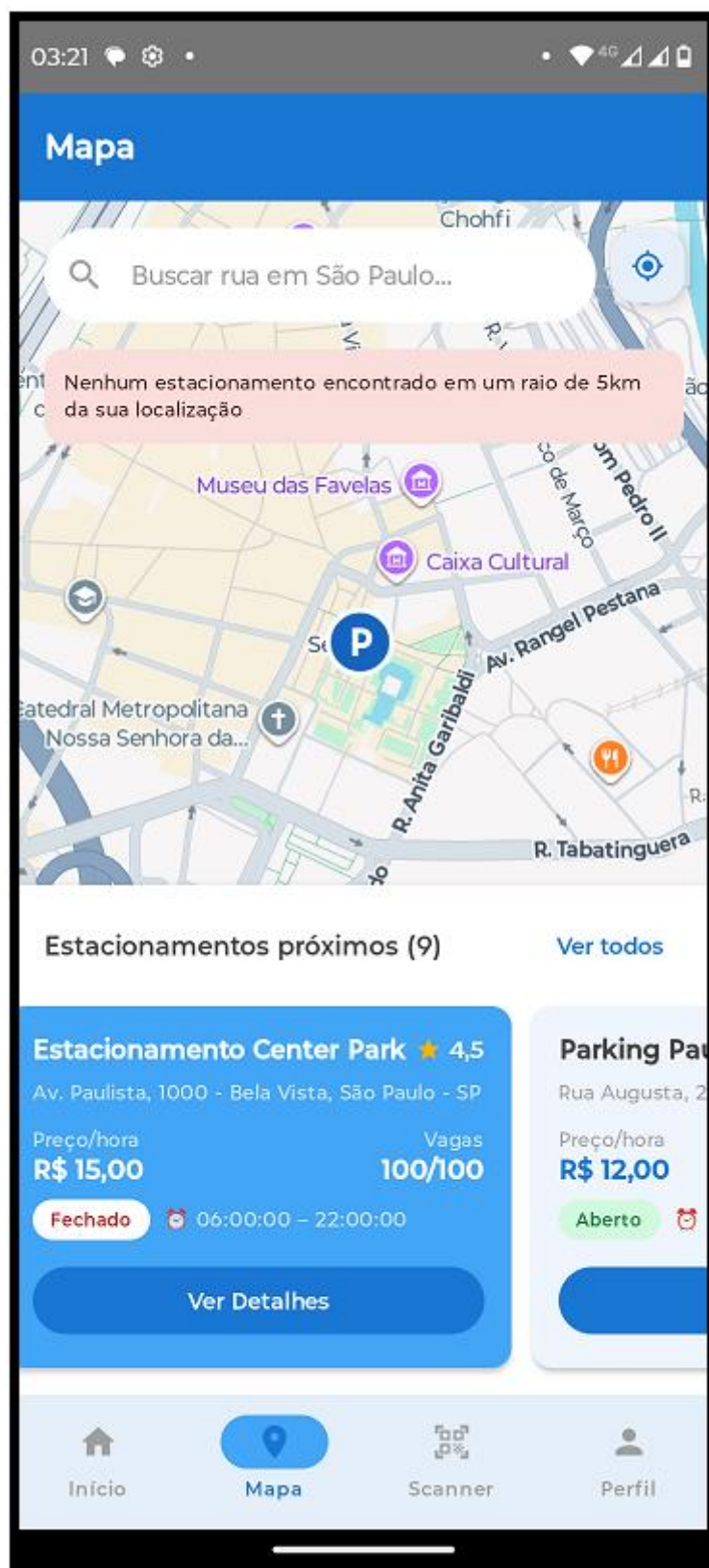
Figura 58 - Mobile - Tela do mapa interativo e os cards dos estacionamentos
