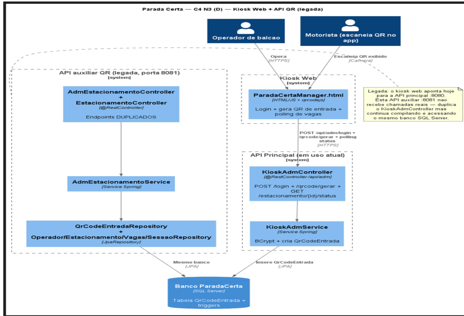
Figura 37 - C4 Nível 3 - QR Code
