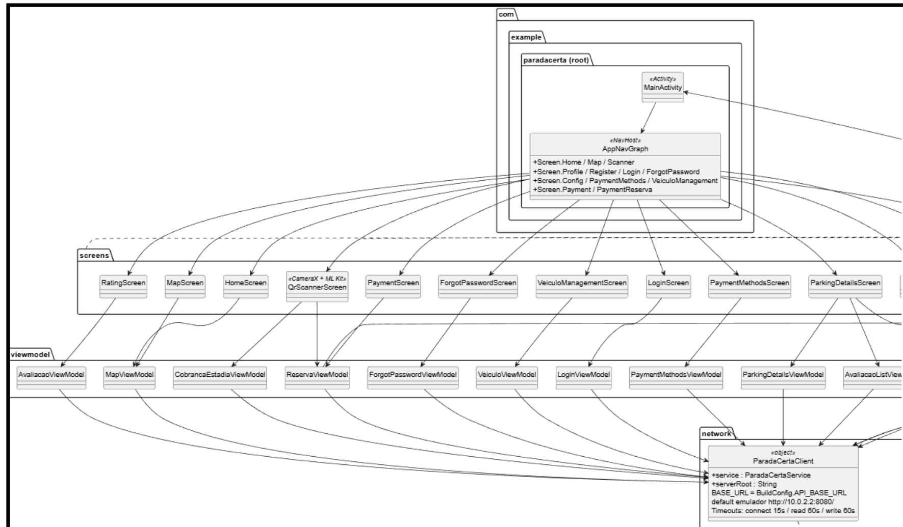
Figura 46 - C4 Nível 4 - ViewModel App (1/2)
