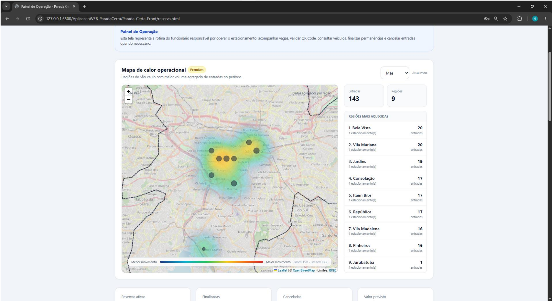
Figura 101 - Web - Painel de Operação (mapa de calor)
