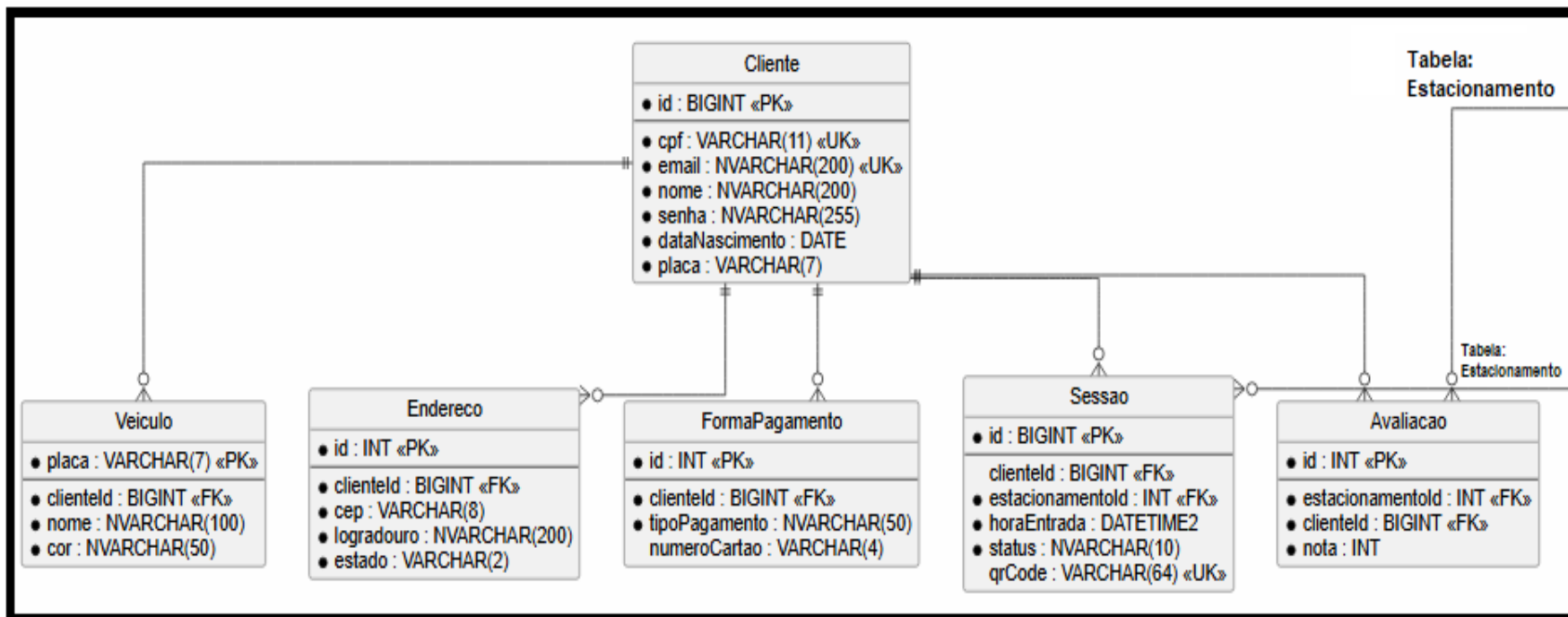
Figura 26 - Diagrama DER (1/2)
