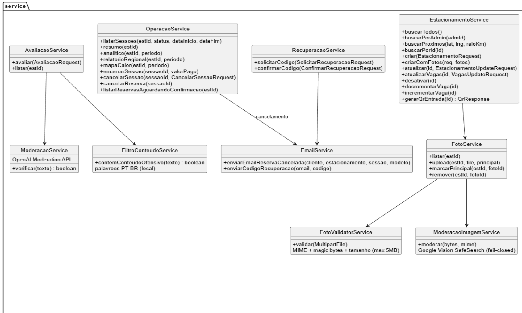
Figura 41 - C4 Nível 4 - Services (2/2)
