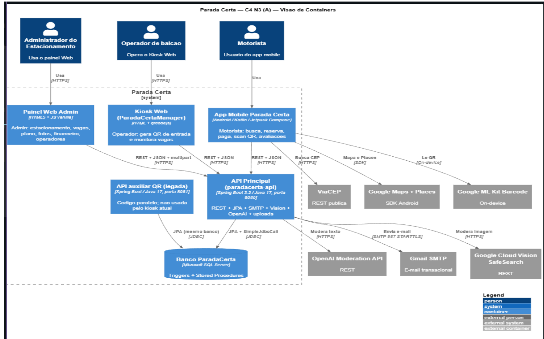
Figura 31 - C4 Nível 3 - Containers
