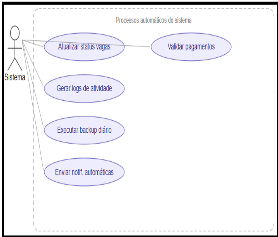
Figura 8 - Diagrama de casos de uso - Parte 3
