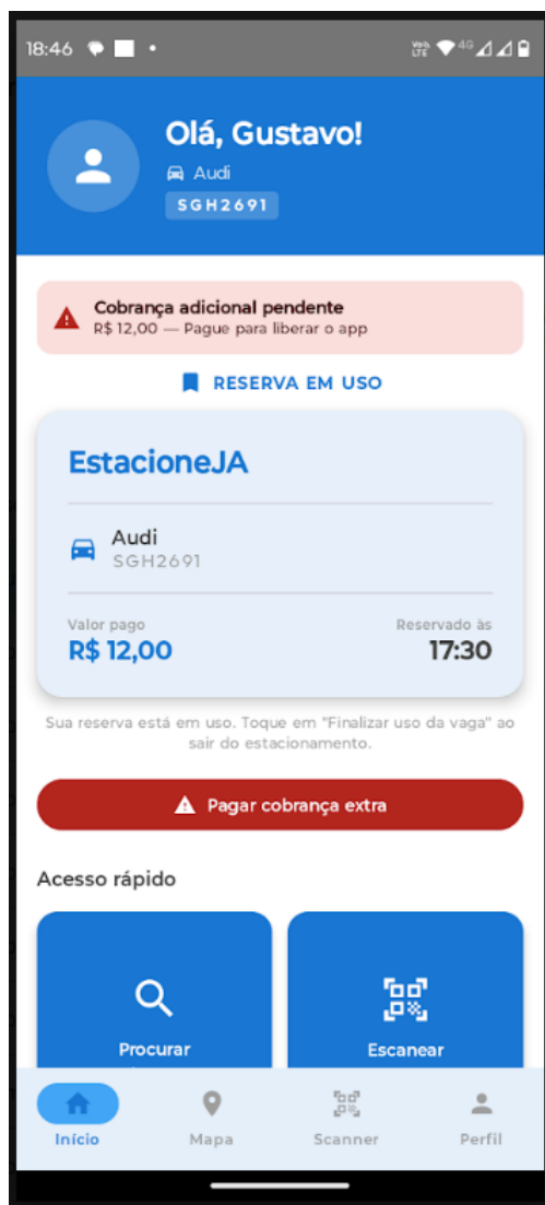
Figura 67 - Mobile - Tela inicial para cobrança extra em reservas
