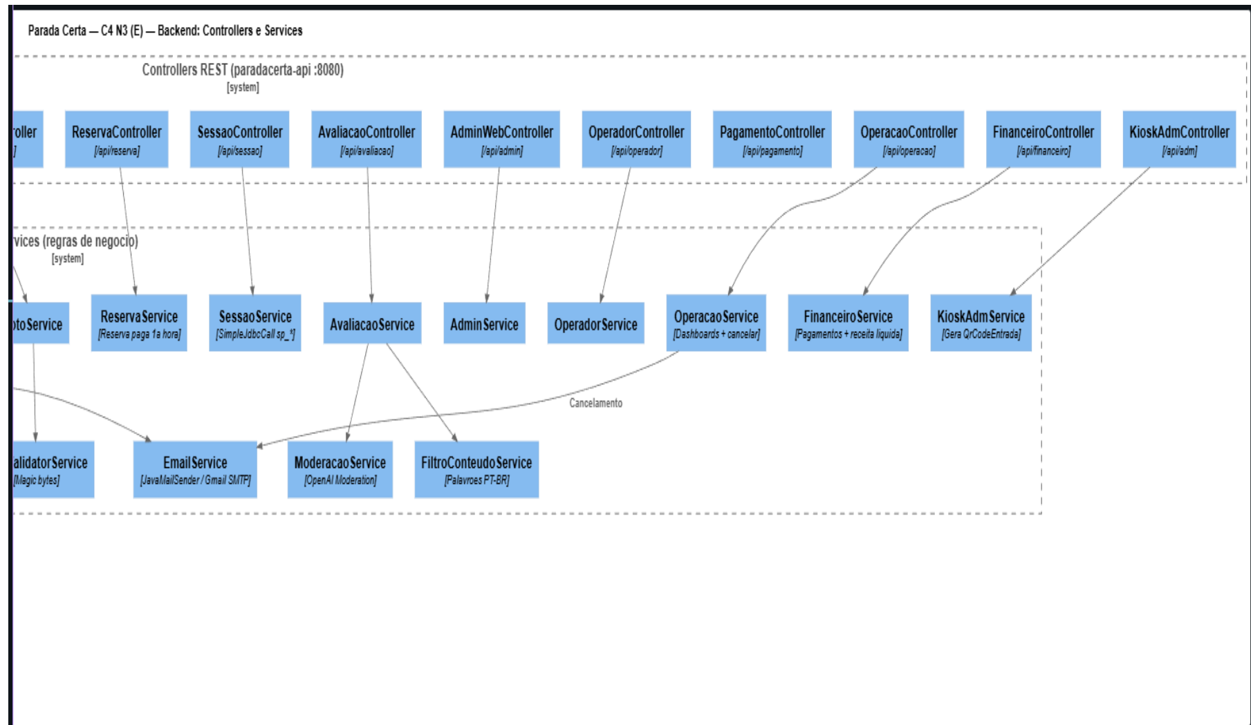
Figura 36 - C4 Nível 3 - Controllers e Services (2/2)
