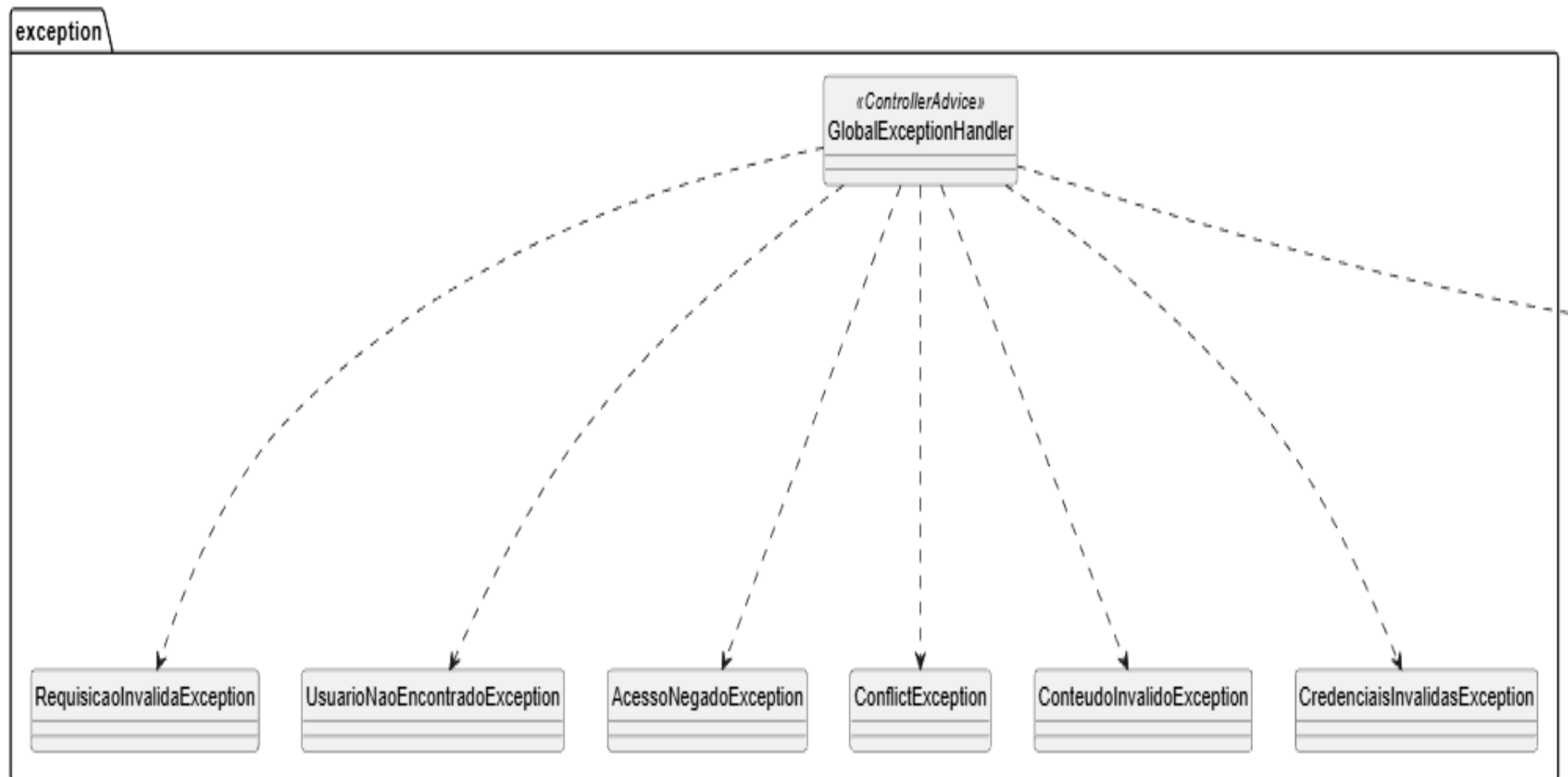
Figura 38 - C4 Nível 4 - Exceptions
