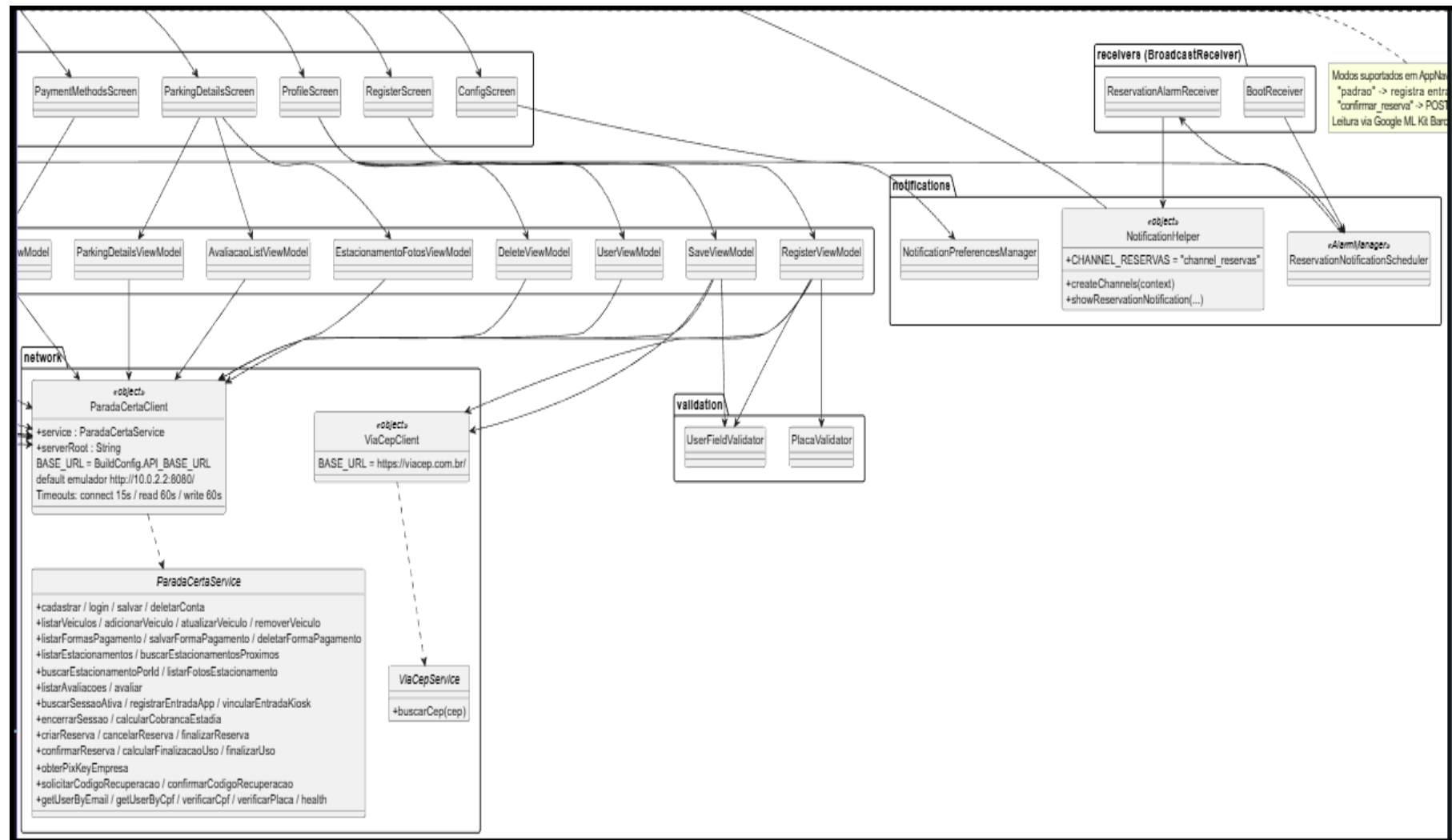
Figura 47 - C4 Nível 4 - ViewModel App (2/2)
