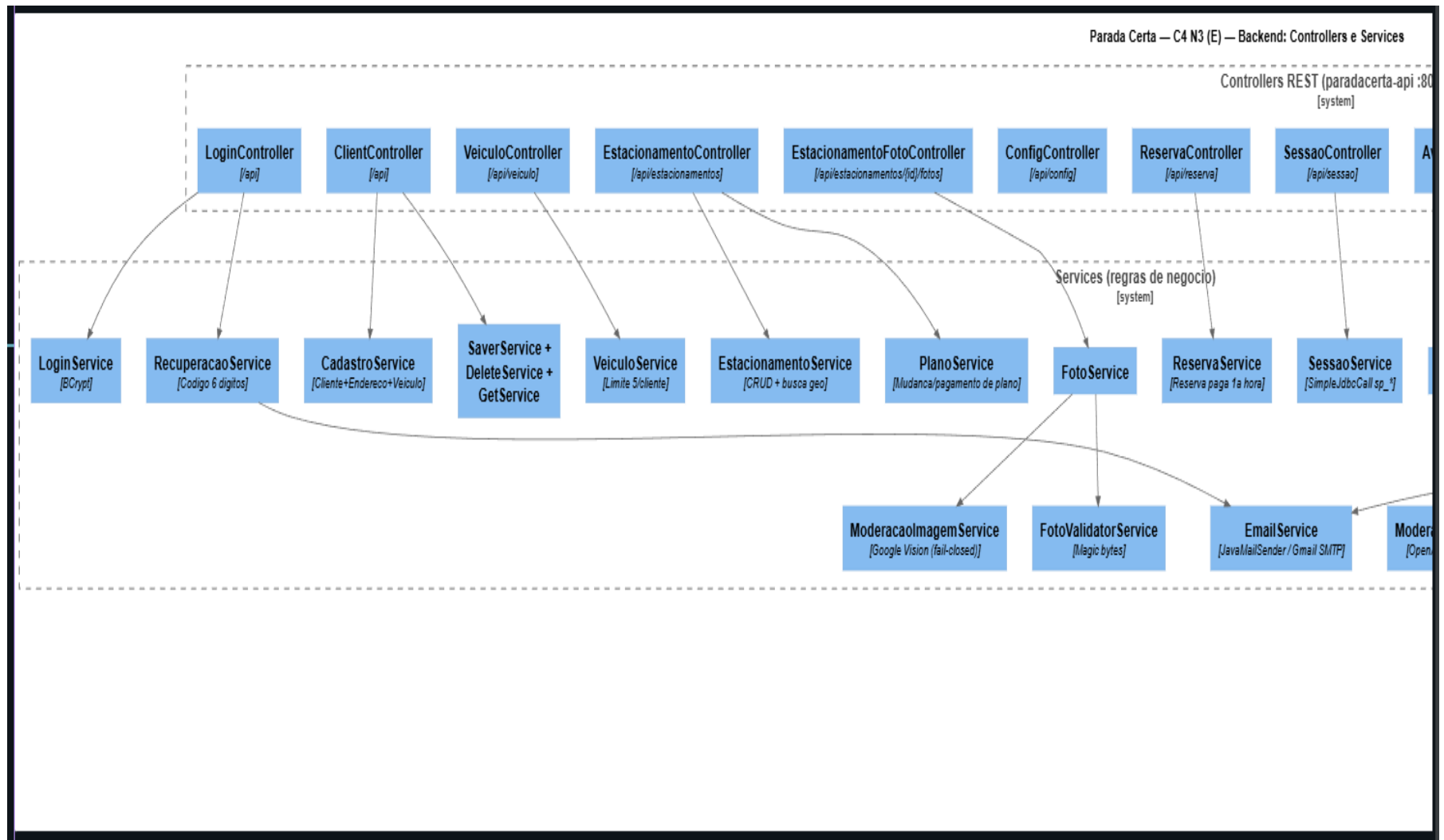
Figura 35 - C4 Nível 3 - Controllers e Services (1/2)
