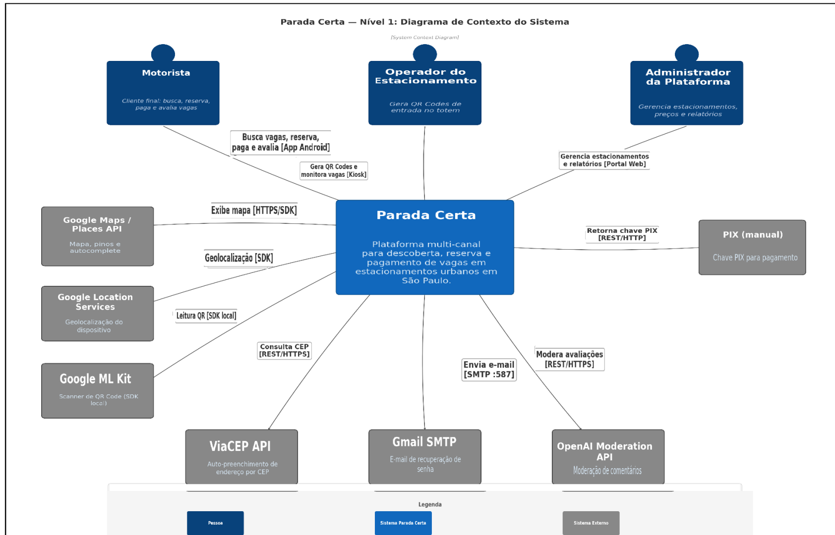
Figura 29 - Diagrama C4 - Nível 1
