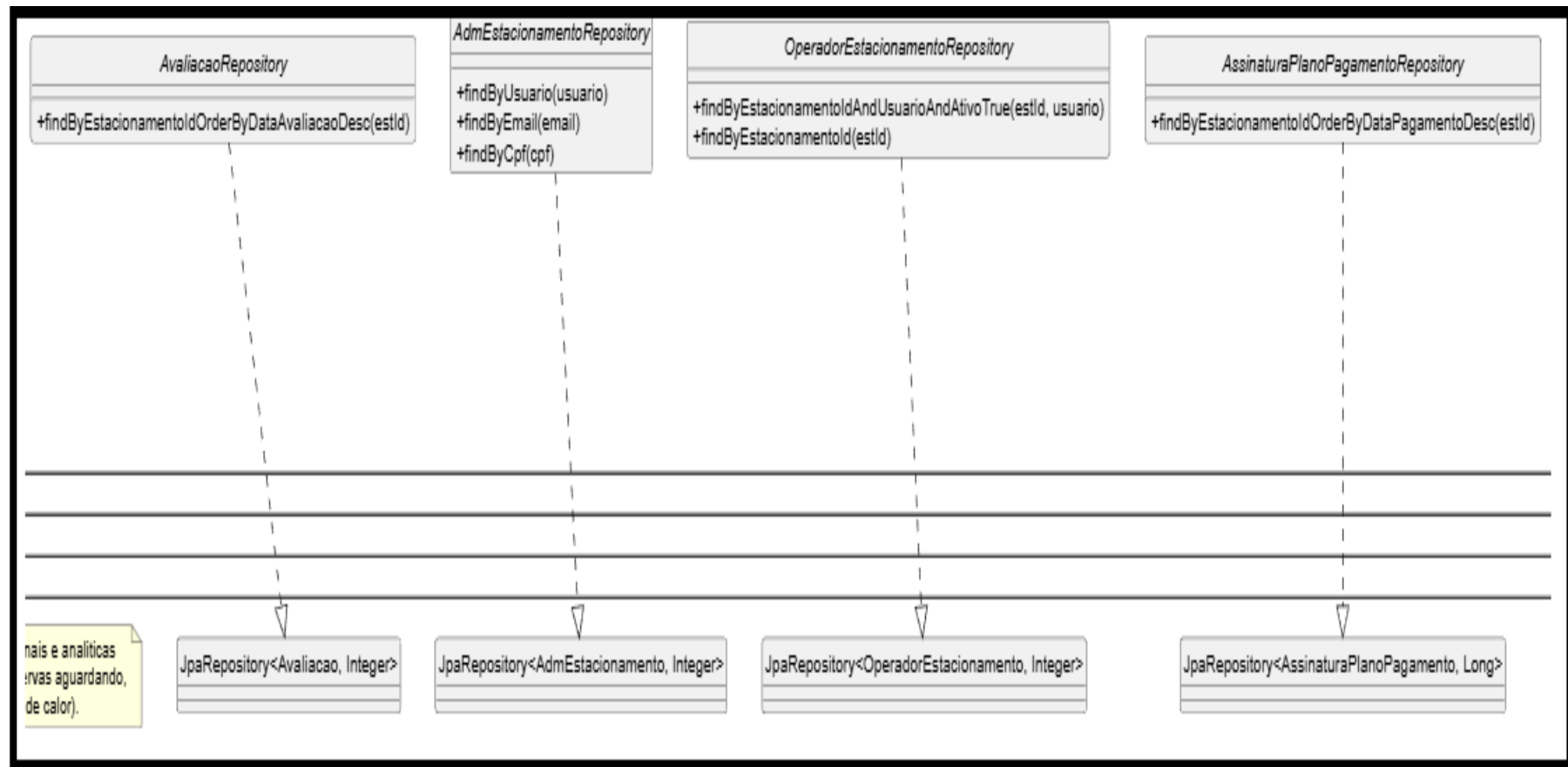
Figura 44 - C4 Nível 4 - Repository (3/3)
