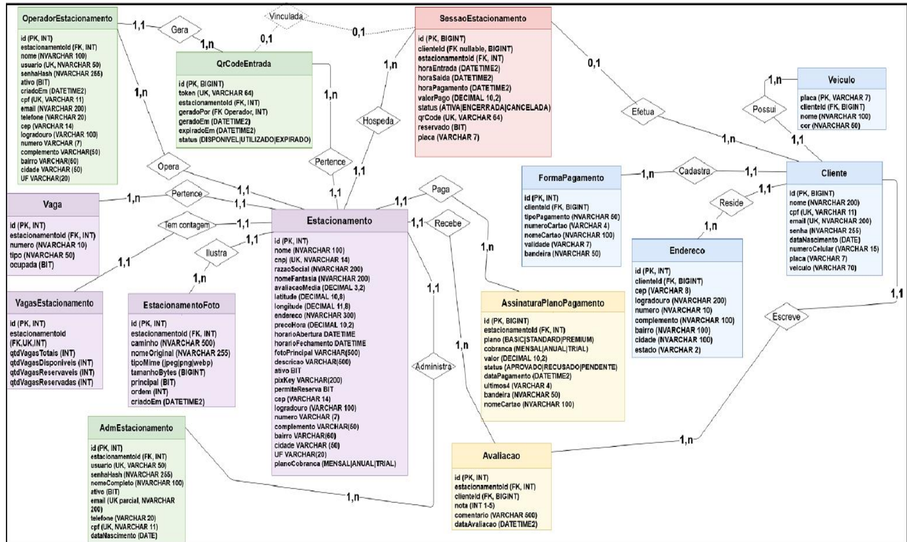
Figura 28 - Modelo físico do banco de dados do sistema
