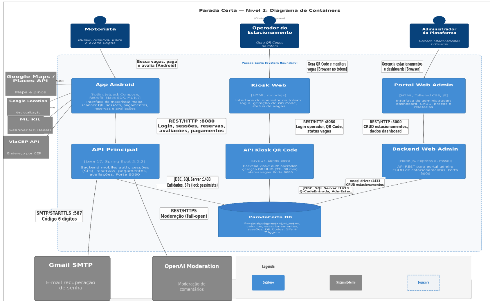
Figura 30 - Diagrama C4 - Nível 2
