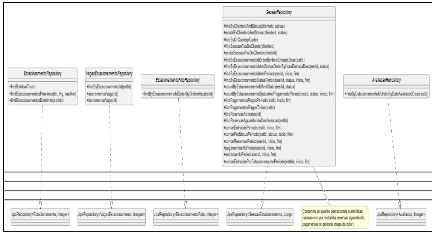
Figura 43 - C4 Nível 4 - Repository (2/3)
