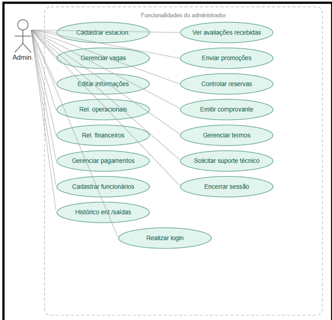
Figura 7 - Diagrama de casos de uso - Parte 2
