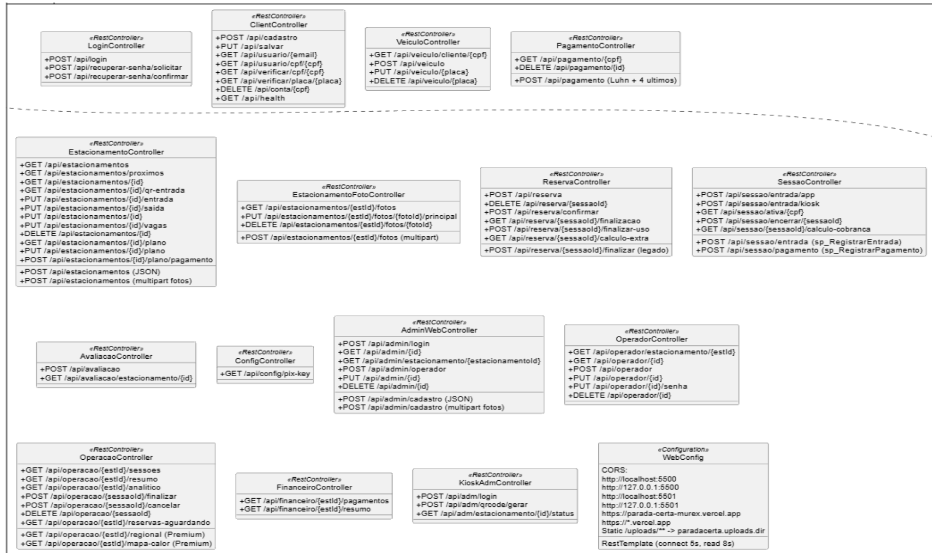
Figura 39 - C4 Nivel 4 - Controllers
